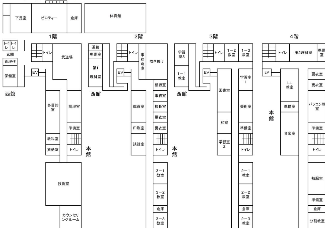
校 舎 配 置 図
