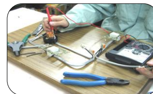
＜電気工事＞
