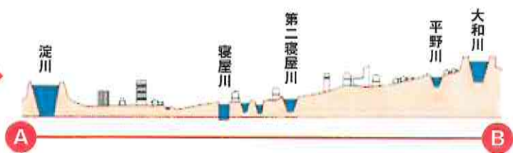
地盤高断面図 (A ~ B 断面)
